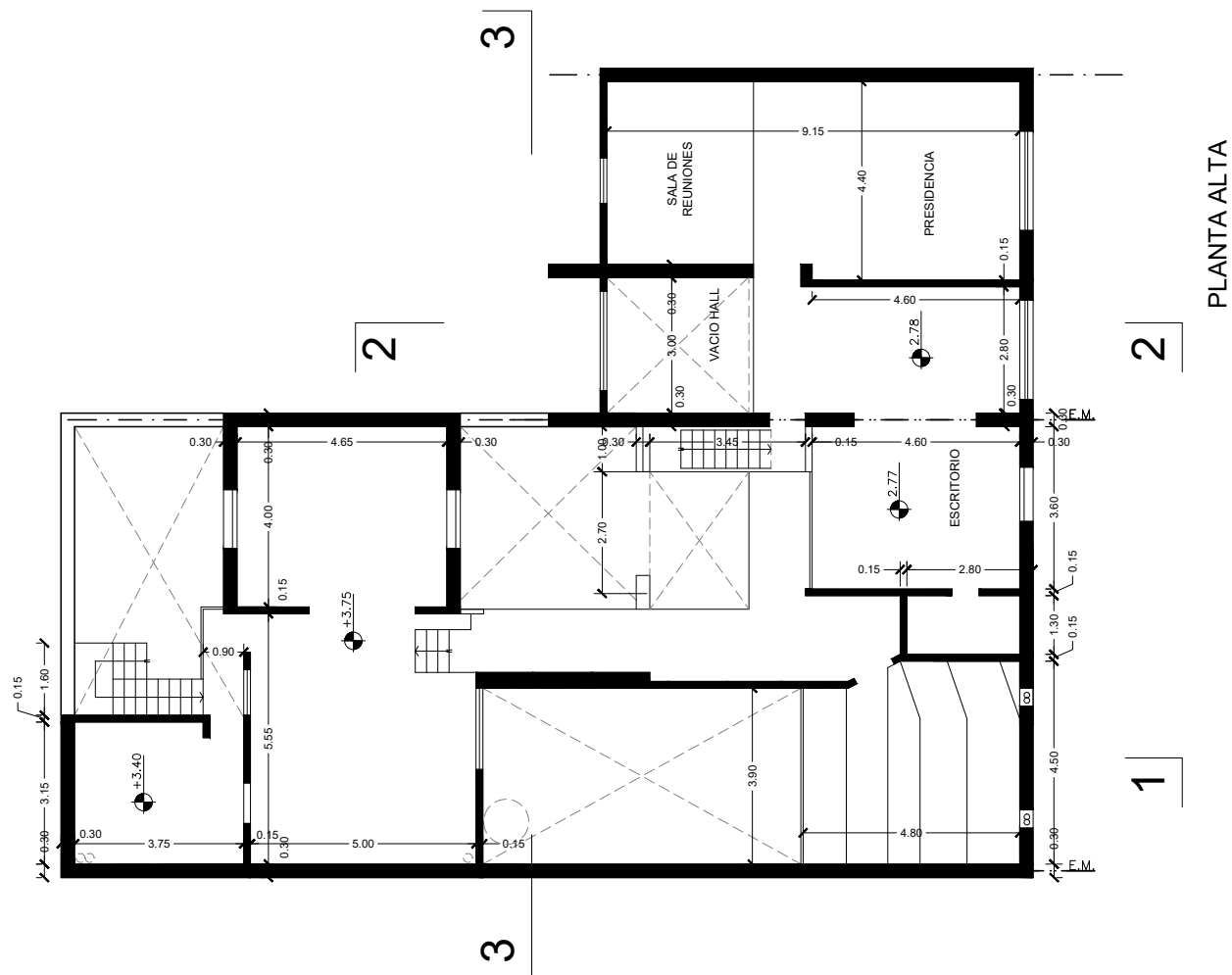
4.7 CAPBAUNO. ESTADO ACTUAL. PLANTA ALTA.
