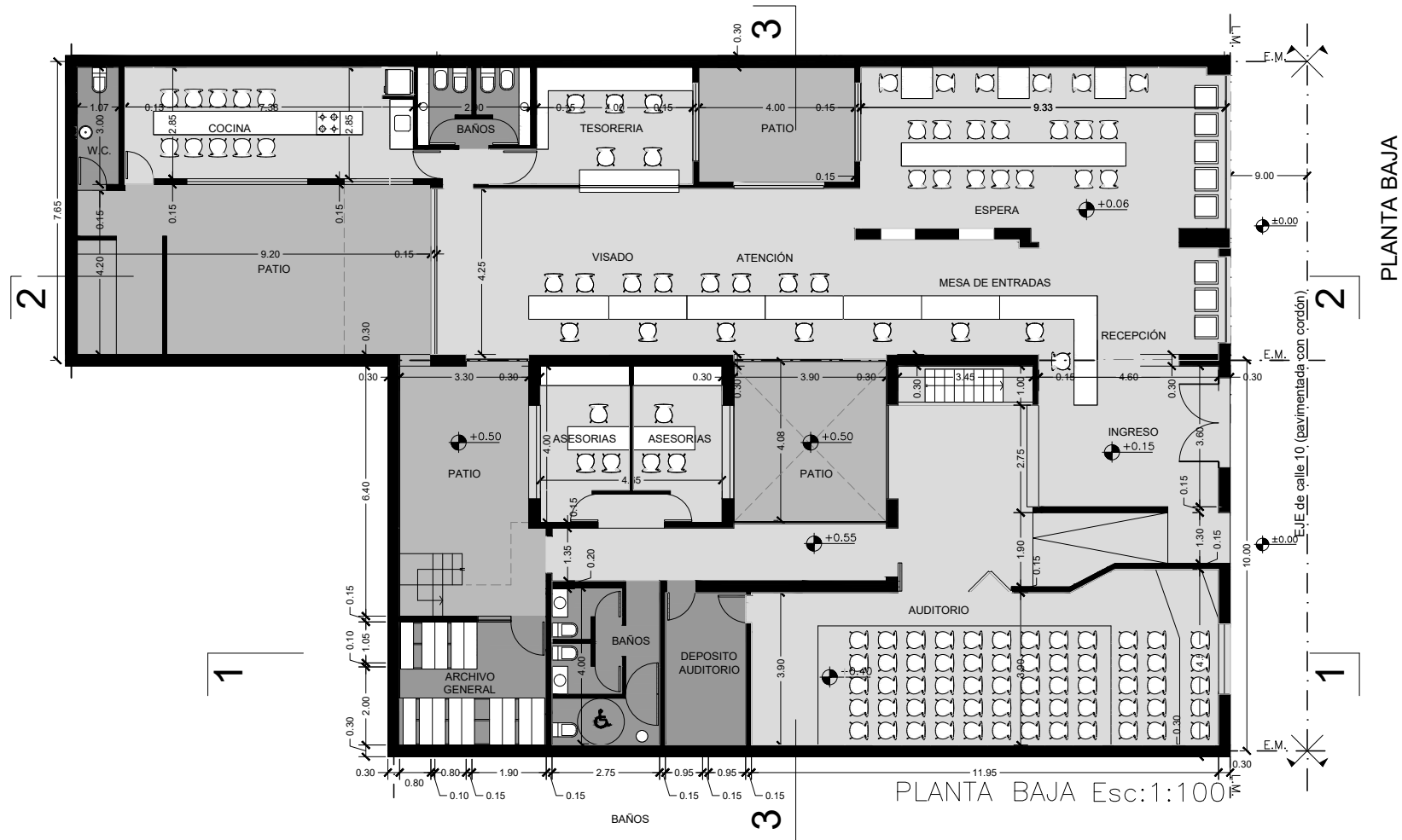
4.7 CAPBAUNO. ESTADO ACTUAL. PLANTA BAJA.
