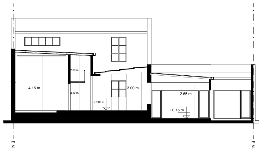
Corte 3-3
